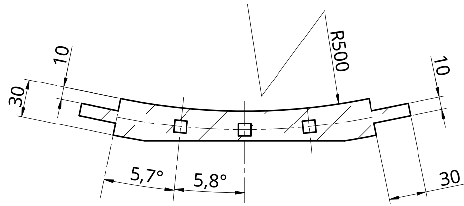
D - D
