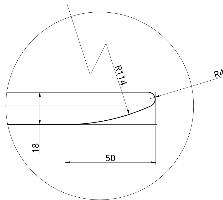
E 1:1
